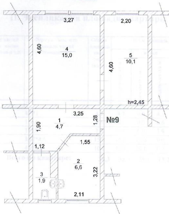
Позтажный план 1 этаж
